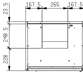
Centrifugal Fan
